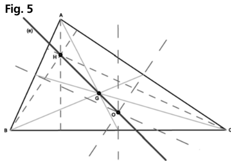
La droite (e) passe par les points de rencontre des hauteurs H, des médianes G et des médiatrices O.
