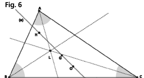
La droite (e) ne passe pas par L (seules les bissectrices apparaissent, les autres familles de droites ont été masquées).
