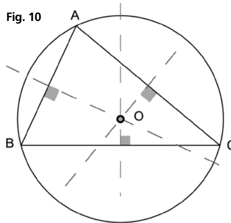
Cercle circonscrit.
