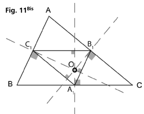
Les médiatrices du triangle A B C sont aussi hauteurs de A_1 B_1 C_1 .
