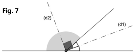
Bissectrice intérieure et extérieure.
